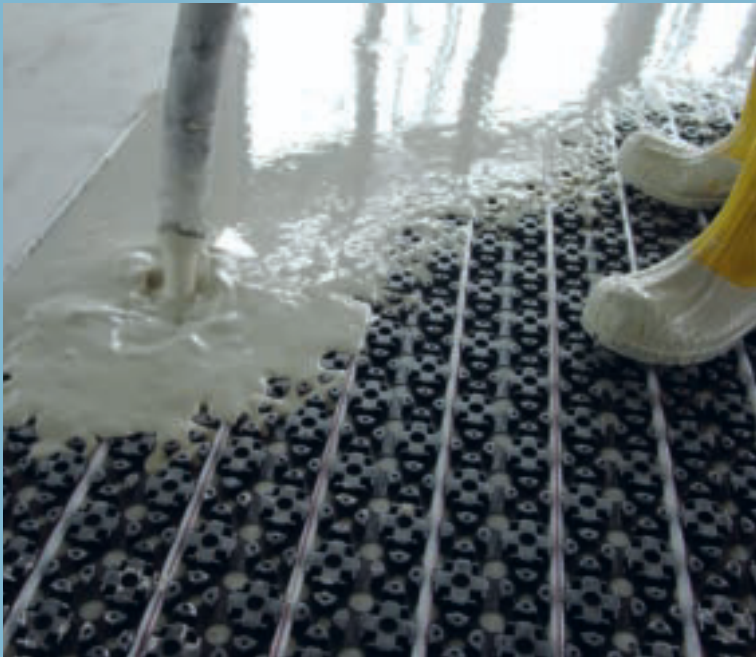
Knauf Nivellierestrich 425 wird auf dem Heizungssystem Uponor Minitec vergossen.
