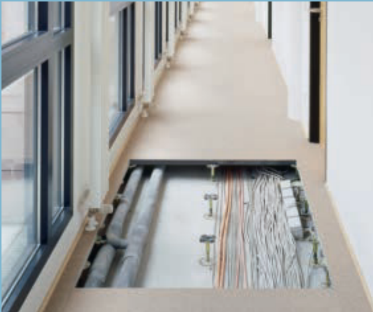
Geöffnete Doppelbodenelemente
