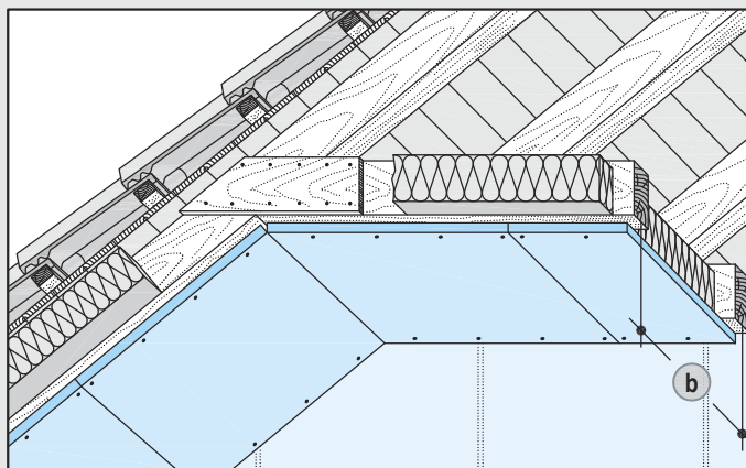
D610 Diamant Direktbekleidung
