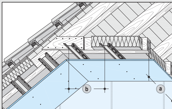
D613 Diamant Metall-Unterkonstruktion Federschiene
